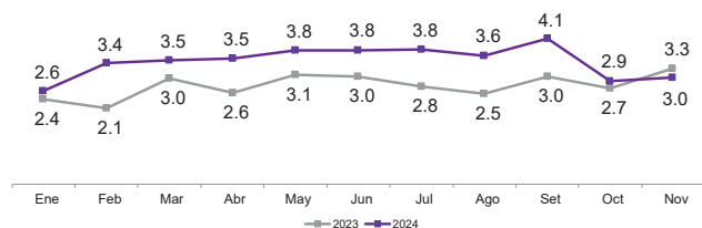
2023 – 2024: Producción mensual de molibdeno (miles de TMF)
