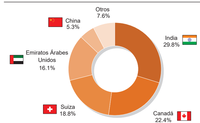
2024: Destino de las exportaciones de oro (enero - octubre)
