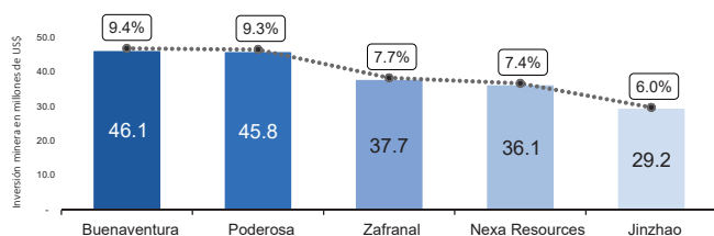
Ranking de inversión minera en Exploración (en millones de US$), enero - noviembre 2024
