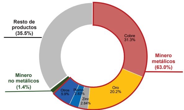
2024: Estructura del valor de las exportaciones (enero-octubre)
