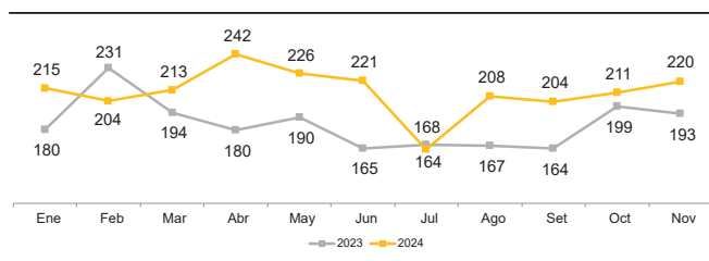
2023 - 2024: Extracción mensual de arena (gruesa/fina) (miles de TM)
