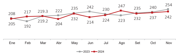
2023 - 2024: Producción mensual de cobre (miles de TMF)
