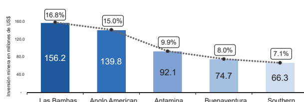
Ranking de inversión minera en Infraestructura (en millones de US$), enero - noviembre 2024
