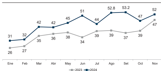
2023 - 2024: Inversión mensual en Exploración (millones de US$)
