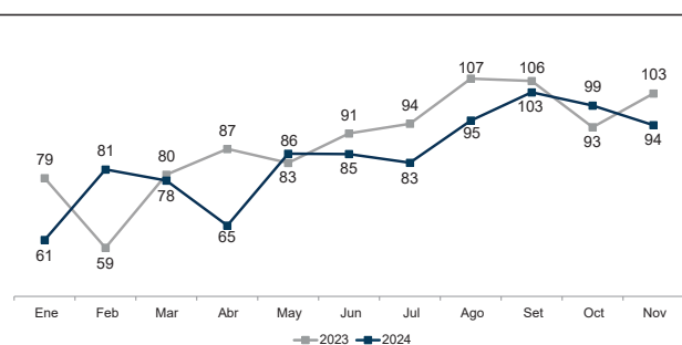
2023 - 2024: Inversión mensual en Infraestructura (millones de US$)
