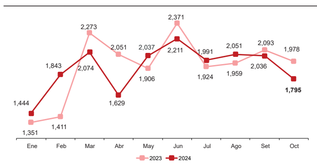
Valor de las Exportaciones de cobre (Valor FOB en millones de US$)
