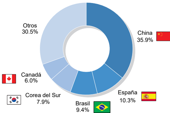
2024: Destino de las exportaciones de zinc (enero - octubre)
