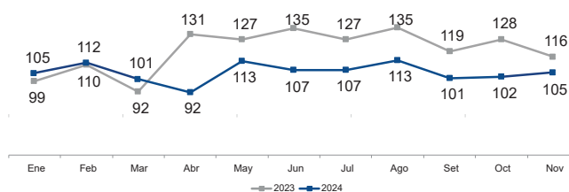
2023 - 2024: Producción mensual de zinc (miles de TMF)
