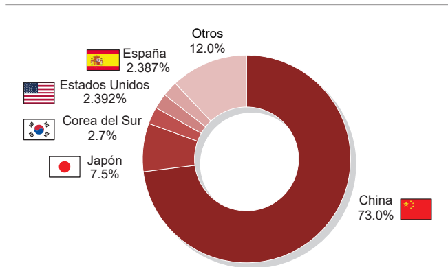
2024: Destino de las exportaciones de cobre (enero - octubre)
