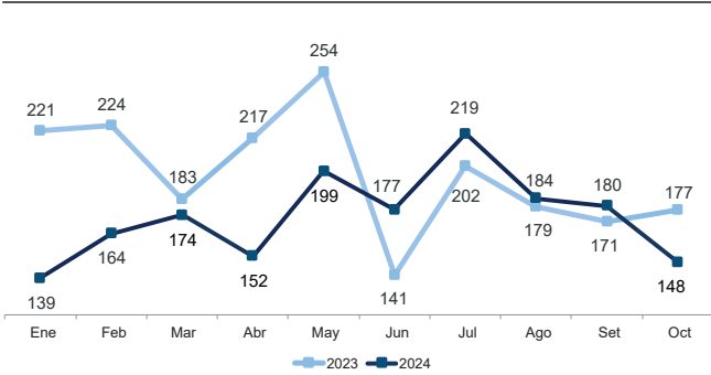
Valor de las Exportaciones de zinc (Valor FOB en millones de US$)
