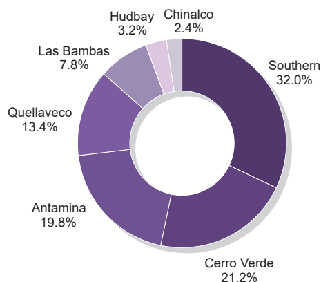
2024: Estructura de la producción de molibdeno por empresas, enero - noviembre
