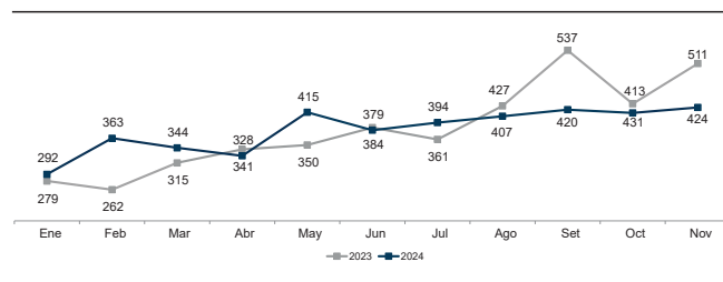
2023 - 2024: Evolución mensual de las inversiones mineras (millones de US$)
