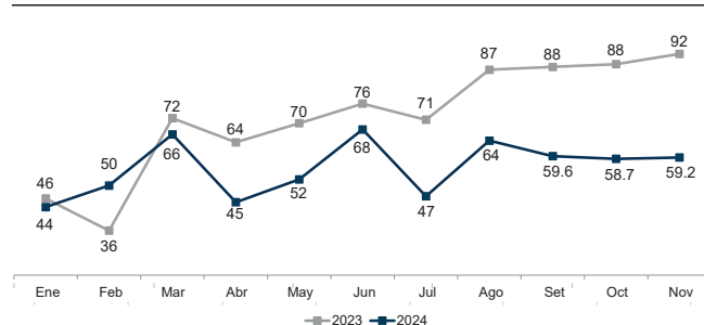
2023 - 2024: Inversión mensual en Desarrollo y Preparación (millones de US$)
