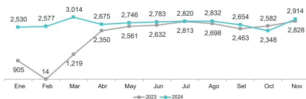
2023 – 2024: Producción mensual de estaño (TMF)
