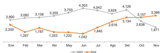
2023 - 2024: Extracción mensual de caliza/dolomita (miles de TM)
