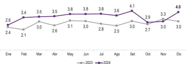
2023 – 2024: Producción mensual de molibdeno (miles de TMF)
